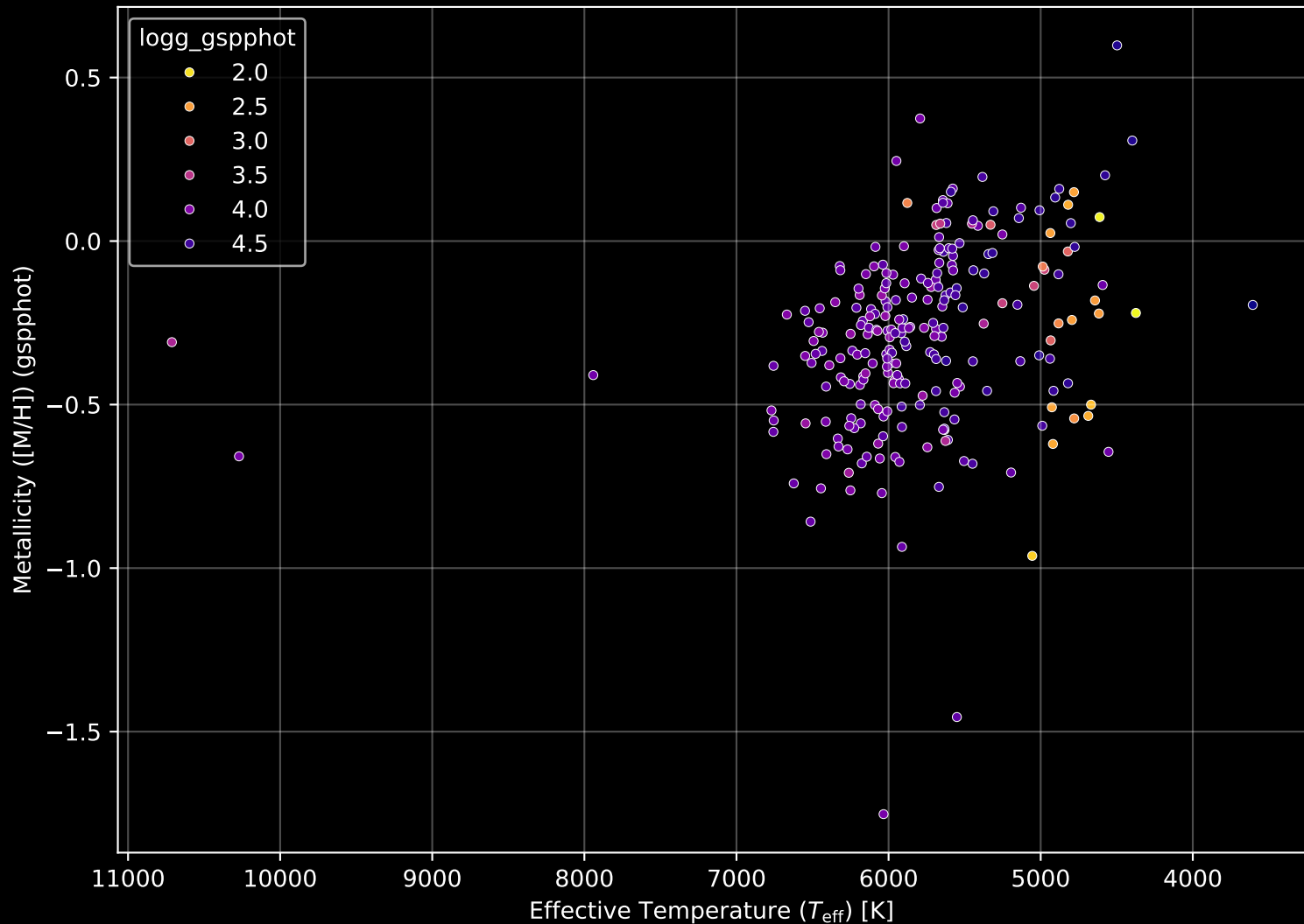
GALAH DR4 Field: [1645] Stellar Population Parameters (n= 245)
