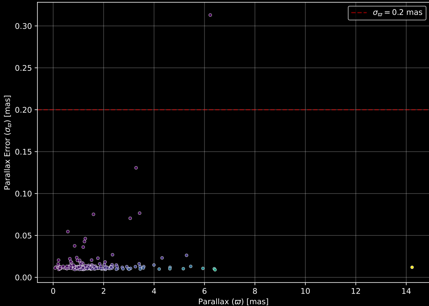
GALAH DR4 Field: [1645] Parallax Quality (n= 245)
