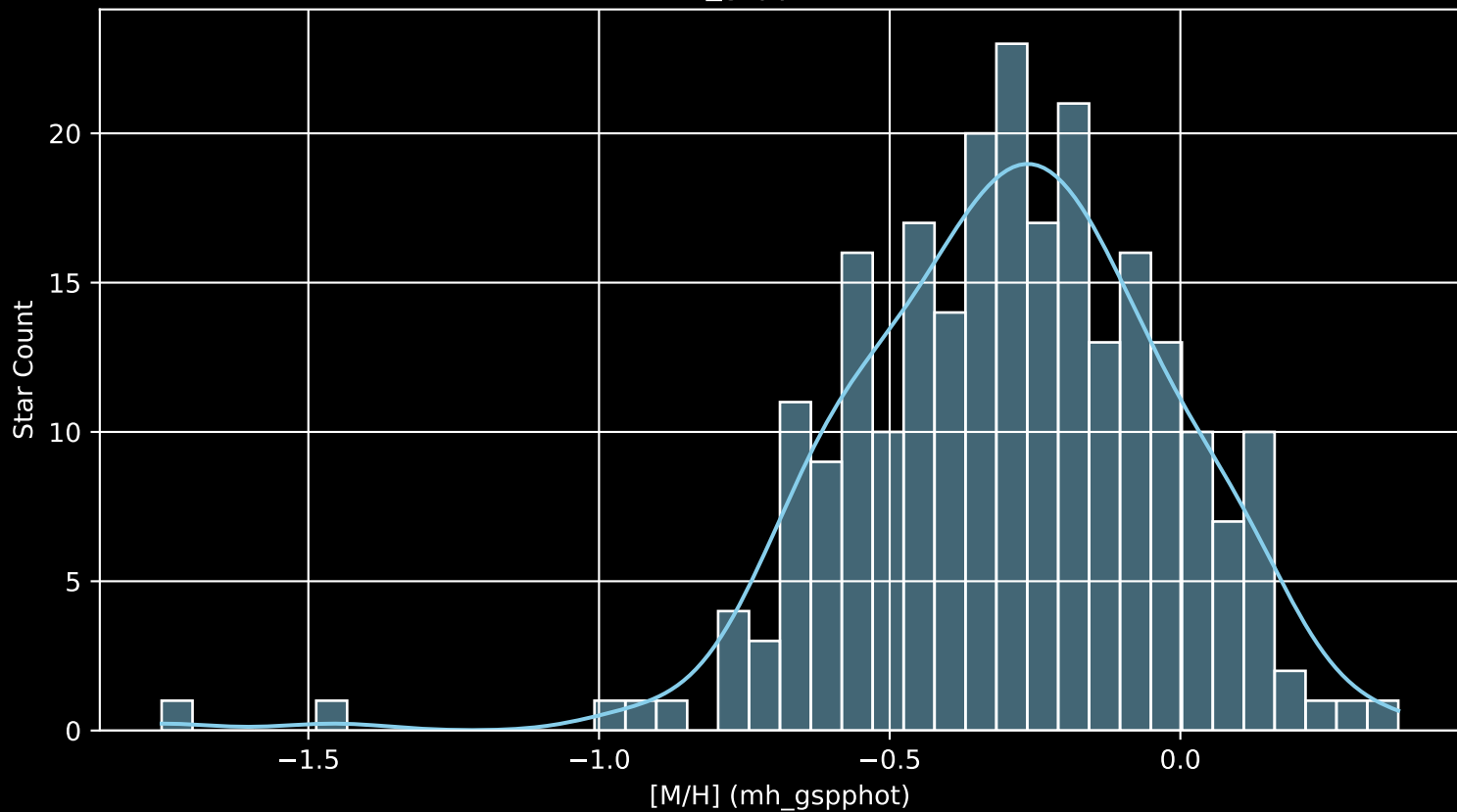
GALAH DR4 Field: [1645] [M/H] (mh_gspphot) (n= 244)
