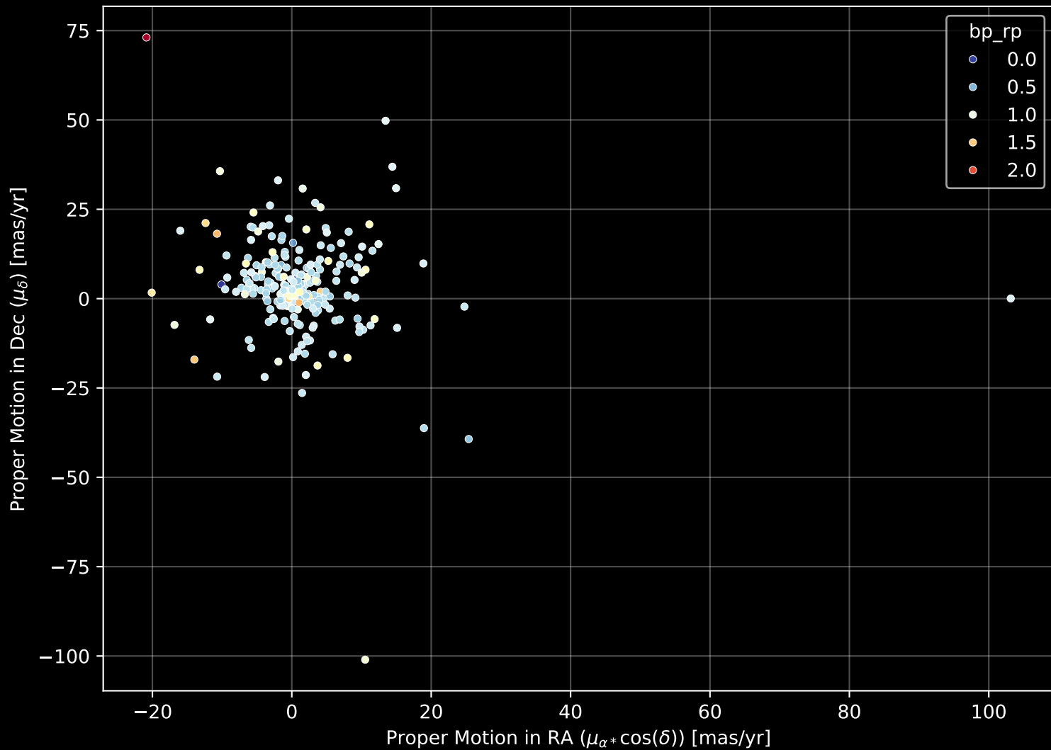
GALAH DR4 Field: [1645] Proper Motion Diagram (n= 245)
